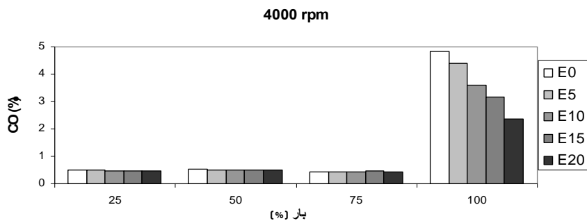
شکل ۴- تاثیر گازول بر مقدار آلاینده CO برای بارهای مختلف موتور در سرعت ۴۰۰۰ دور بر دقیقه
