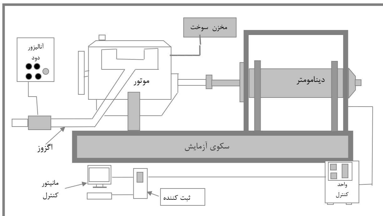
شکل ۱- شماتیک سکوی آزمایش موتور
