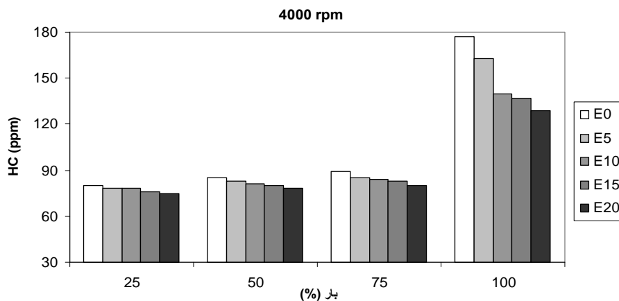
شکل ۸- تاثیر گازول بر مقدار HC برای بارهای مختلف موتور در سرعت ۴۰۰۰ دور بر دقیقه
