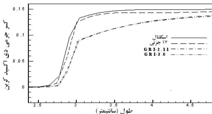
شکل ۱۱- توزیع جزء جرمی دی اکسید کربن با استفاده از چهار سازوکار متفاوت در حالت استوکیومتریکی و در حالت بزرگنمایی
