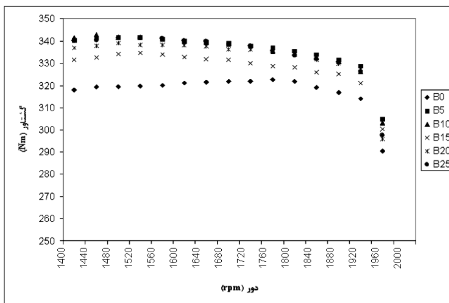
شکل ۲- رابطه‌ی بین گشتاور - دور برای ترکیبات مختلف سوخت دیزل - بیودیزل
