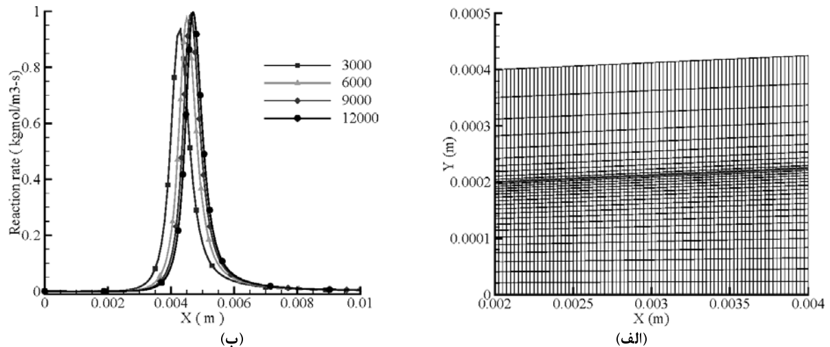
شکل 2- الف) بخش بزرگنمایی شده از شبکه بندی مورد استفاده (ب) نمودار تغییرات نرخ پیشرفت واکنش در میکروبرنر
