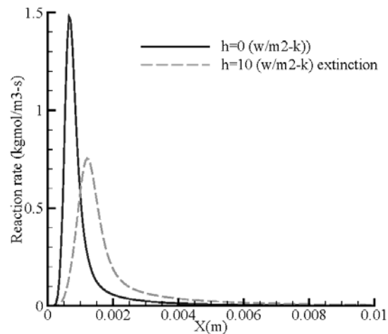
شکل 6- پدیده‌ی خفگی - نرخ انجام واکنش در محور تقارن برای کانالی با زاویه انحراف 0/7 درجه در حالت k_{\text{wall}}=15\text{W/mK} , v=0/5\text{m/s} و h=10\text{W/m}^2\text{K}
