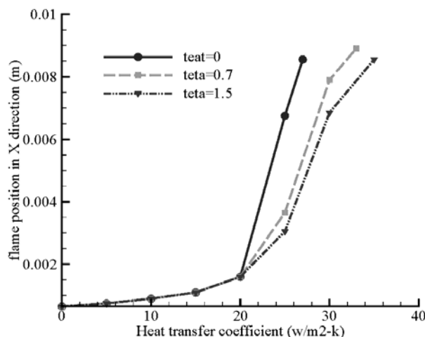
شکل 12- مکان شعله بر حسب ضریب انتقال حرارت جابجایی برای سه زاویه مختلف در v=1\text{m/s} و k_{\text{wall}}=1\text{W/mK}
