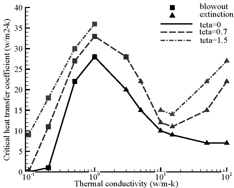
شکل 13- ضریب انتقال حرارت بحرانی بر حسب ضریب انتقال حرارت رسانشی دیواره در سه زاویه‌ی مختلف با سرعت ورودی 0/5 متر بر ثانیه
