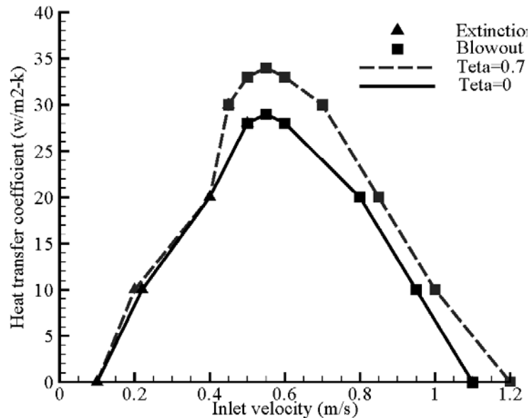
شکل 14- نقشه‌ی پایداری- محدوده‌ی سرعت بر حسب ضریب انتقال حرارت جابجایی دیواره در k_{wall}=1W/mK برای کانال مستقیم و کانال واگرا با زاویه‌ی 0/7 درجه
