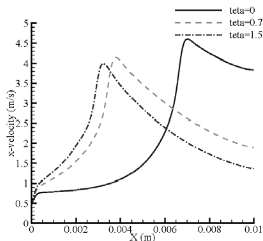
شکل 8- نمودار سرعت در راستای محور x در محور تقارن با سه زاویه‌ی متفاوت در حالتی که v=5\text{m/s} , h=25\text{W/m}^2\text{K} , k_{\text{wall}}=1\text{W/mK}
