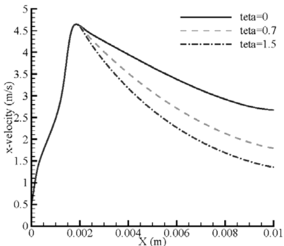
شکل 7- نمودار سرعت در راستای محور x در محور تقارن با سه زاویه‌ی متفاوت در حالتی که h=20\text{W/m}^2\text{K} , k_{\text{wall}}=1\text{W/mK} , v=0/5\text{m/s}
