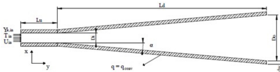
شکل 1- شکل شماتیک میکرو برنر مورد بررسی
