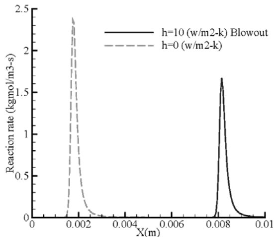
شکل 5- پدیده‌ی خروج شعله از کانال - نرخ انجام واکنش در محور تقارن برای کانالی با زاویه انحراف 0/7 درجه در حالت v=0/5\text{m/s} و h=10\text{W/m}^2\text{K} , k_{\text{wall}}=0/2\text{W/mK}
