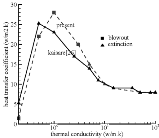
شکل 3- مقایسه نتایج پروژه‌ی حاضر با پژوهش [7] برای مخلوط پروپان-هوا با سرعت ورودی v=0.5\text{m/s} در کانال مستقیم به عرض 400\mu\text{m} و ضخامت دیواره 200\mu\text{m}
