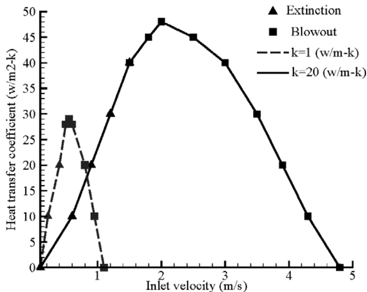
شکل 15- نقشه‌ی پایداری - محدوده‌ی سرعت بر حسب ضریب انتقال حرارت جابجایی دیواره برای کانال مستقیم با دو ضریب رسانشی k_{wall}=20W/mK و k_{wall}=1W/mK
