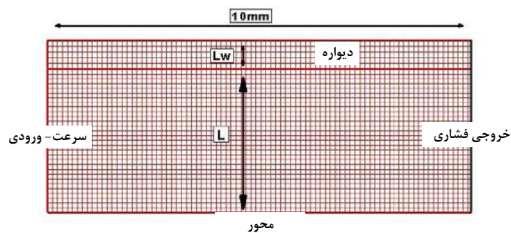
شکل ۴- نمایش هندسه تقارن محوری محفظه احتراق به همراه شبکه تولید شده
