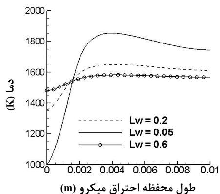
شکل ۱۴- نمودار توزیع دما بر روی دیواره محفظه احتراق برای سه ضخامت مختلف ( L_w: 0.05, 0.2, 0.6 \text{ mm} ) ( L = 2 \text{ mm} ; K_w = 7.5 \text{ W/m.K} ; V_{in} = 0.2 \text{ m/s} ; h_{out} = 8 \text{ W/m}^2.\text{K} )
