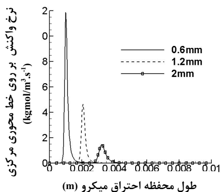
شکل ۱۳- نمودار توزیع نرخ واکنش در مرکز محفظه احتراق برای سه ارتفاع مختلف (L: 0.6, 1.2, 2 mm) ( K_w = 7.5 \text{ W/m.K} ; V_{in} = 0.5 \text{ m/s} ; h_{out} = 0 \text{ W/m}^2.\text{K} )
