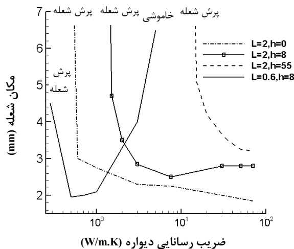
شکل ۱۰- نمودار مکان شعله بر حسب رسانایی دیواره برای سه مقدار ضریب انتقال گرمای جابه‌جایی خارجی ( h=h_{out}: 0, 8, 55 \text{ W/m}^2.\text{K} ) و دو عرض متفاوت محفظه احتراق ( L: 0.6, 2 \text{ mm} ) در V_{in} = 0.3 \text{ m/s}
