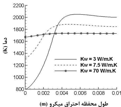
شکل ۹- توزیع دمای دیواره در امتداد طول برای رسانایی‌های مختلف ( K_w: 3, 7.5, 70 \text{ W/m.K} ) ( L = 12 \text{ mm} ; V_{in} = 0.5 \text{ m/s} ; h_{out} = 8 \text{ W/m}^2.\text{K} )
