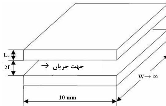
شکل ۳- نمایش هندسه محفظه احتراق میکروکانالی مدل‌سازی شده
