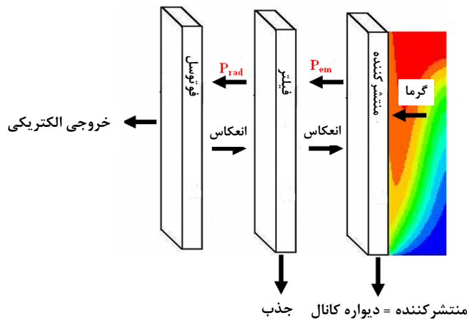
شکل ۲- طرحواره کلی از نحوه تولید توان در یک سامانه میکروترموپوفوتولتائیک
