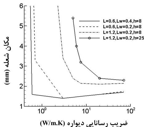
شکل ۱۱- نمودار مکان شعله بر حسب رسانایی دیواره برای ( L : 0.6, 1.2 mm)، ( L_w : 0.2, 0.4 mm) و ( h=h_{out} : 8, 25 W/m 2 .K) در V_{in} = 0.5 m/s
