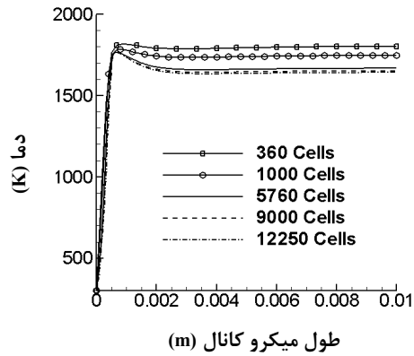
شکل ۵- فرآیند مطالعه شبکه‌بندی مناسب میدان
