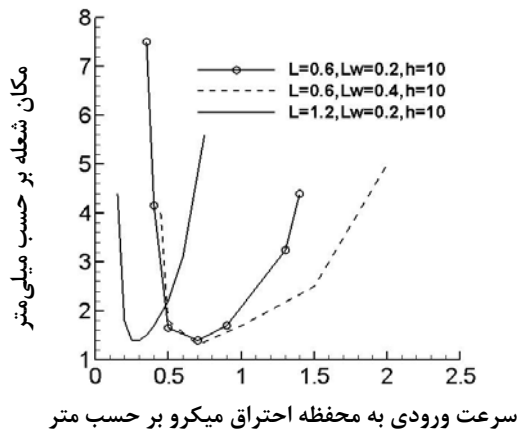
شکل ۱۷- تغییرات مکان شعله بر حسب سرعت ورودی (L: 0.6, 1.2 mm; L w : 0.2, 0.4 mm; h out : 10 W/m 2 .K; K w : 7.5 W/m.K)
