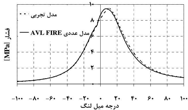
شکل ۳- مقایسه منحنی فشار متوسط داخل سیلندر با نتایج تجربی برای حالت موتور پایه بر حسب درجه میل‌لنگ
