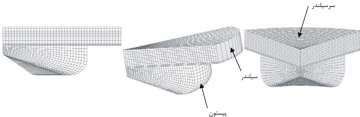
شکل ۱- شبکه محاسباتی برای حالت پایه در زاویه ۲۰ BTDC
