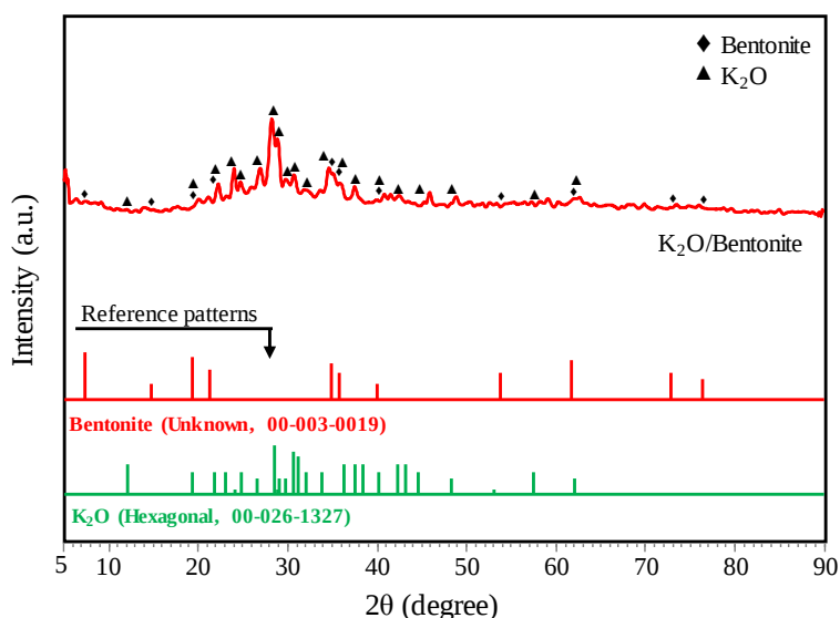
Figure 3- XRD analysis of sonochemically-prepared \text{K}_2\text{O} /Bentonite nanocatalyst شکل ۳- آزمون XRD نانوکاتالیزور \text{K}_2\text{O} /Bentonite تهیه‌شده به روش امواج فراصوت شیمیایی
